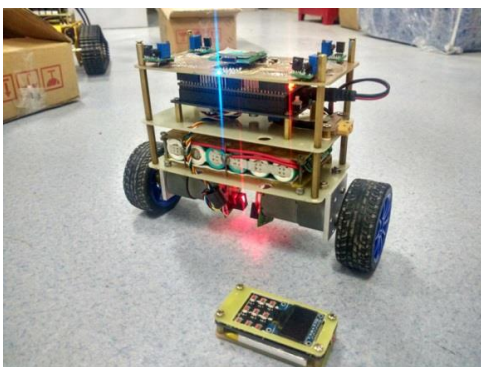
我系参赛作品——两轮自平衡小车
